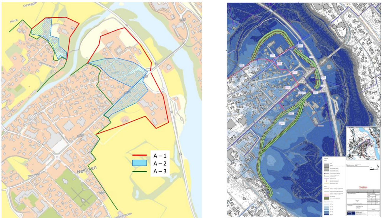
Figur 1 Oversikt over trase alternativer flomvoll Nesflata, fra mulighetsstudie t.v. og forprosjektrapporten t.h.
