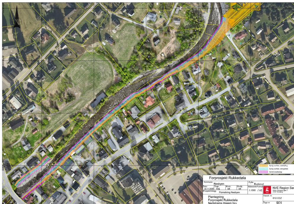
Figur 5. Oversikt over område for sikring av Rukkedøla nedstrøms Hajem bru
