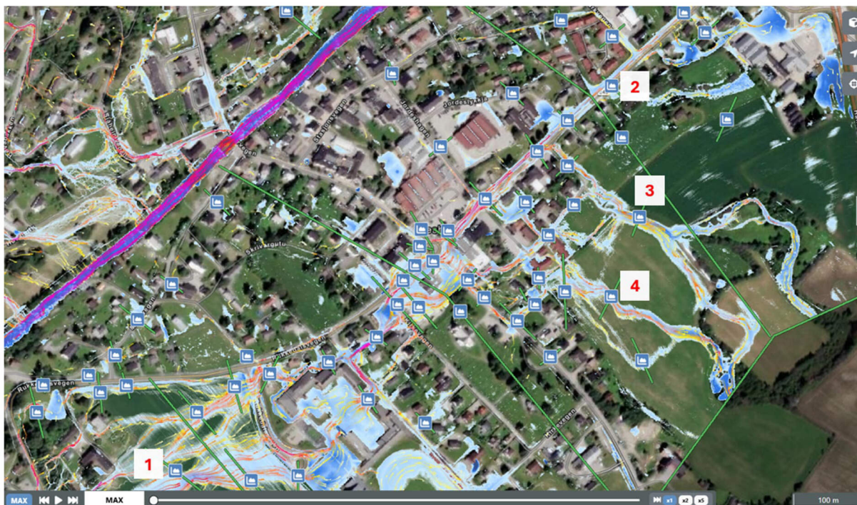
Figur 4.2 Utklipp av resultatene fra simulering av avrenningen for eksisterende tilstand, nedre del av nedbørfeltet, nedbørhendelse N200+klime/D180min.
