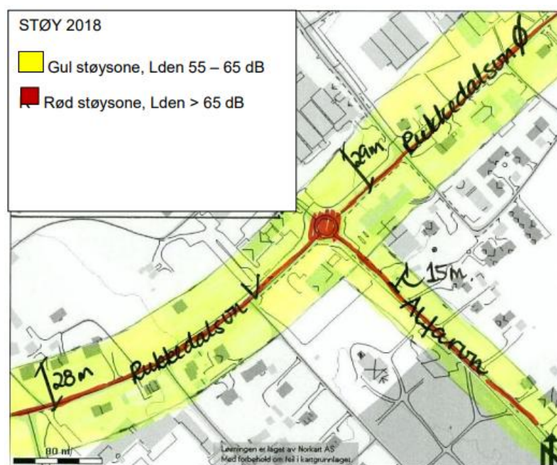
Figur 21. Prinsipp for støysonekart langs Rukkedsalsveien og Alfarseien. Støykoter er tegnet
