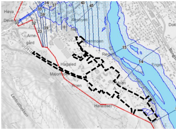
Figur 17. Faresonekart (NVE Atlas) som viser fare for flom (200 års) med blå skravur. Svart stiple linje viser plangrense.
